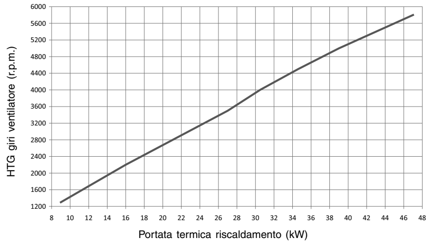
Curva portata termica - nr. giri ventilatore (Qn risc ) Power Green 50
