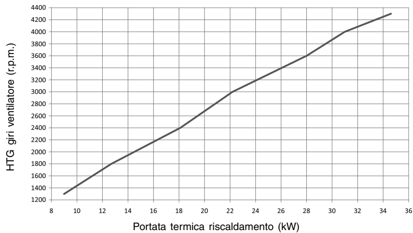
Curva portata termica - nr. giri ventilatore (Qn risc ) Power Green 50 DEP
